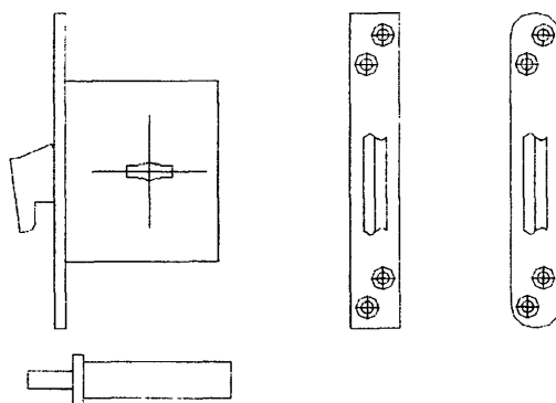
Рисунок Б.4 — Пример замка с крюкообразным засовом
